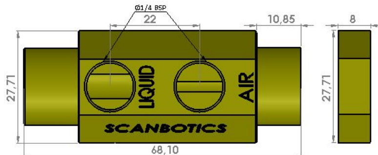
ADAPTATEUR REF : ADAPT.2TLEC
