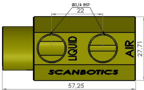
ADAPTATEUR REF : ADAPT.2TL
