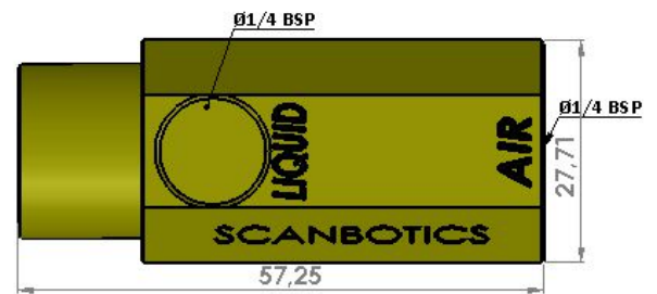
ADAPTATEUR REF : ADAPT.1TL
